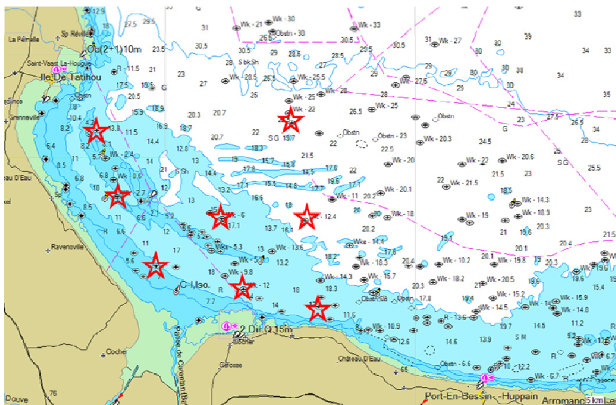
Figure 11 : Proposition d'épaves pour un réseau d'écouteurs en BSO pendant la phase 2.
