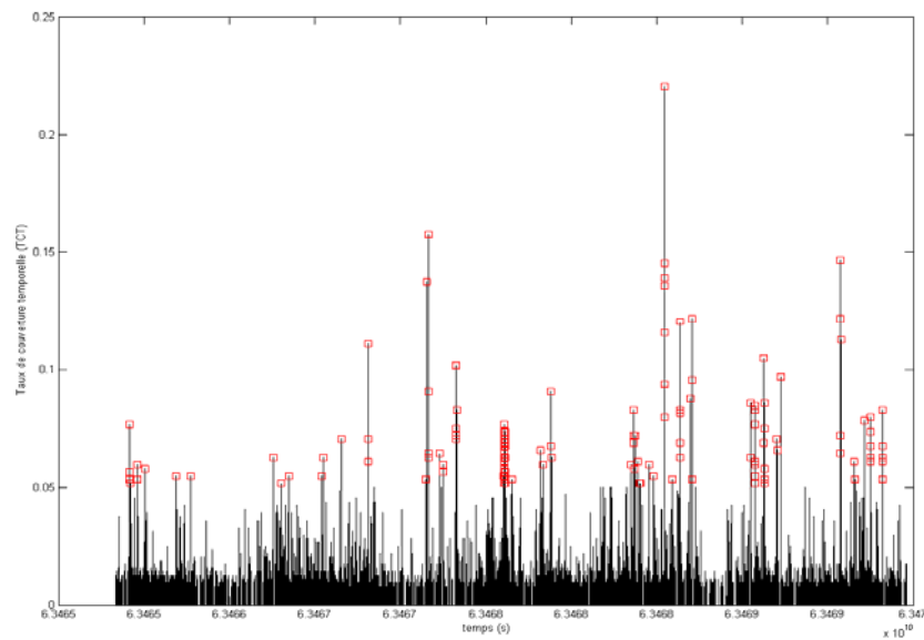
Figure 5 : Taux de couverture temporelle (pics noirs) et détections retenues pour l'identification (carrés rouges).
