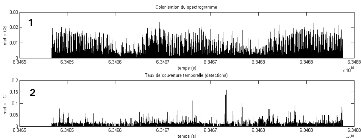
Figure 4.1) Taux de colonisation du spectrogramme (CS) pendant toute la durée de l'enregistrement, comprenant tous les événements énergétiques détectés, et 2) taux de couverture temporelle, comprenant les événements énergétiques après filtrage et seuillage et correspondant aux signaux d'intérêt.
