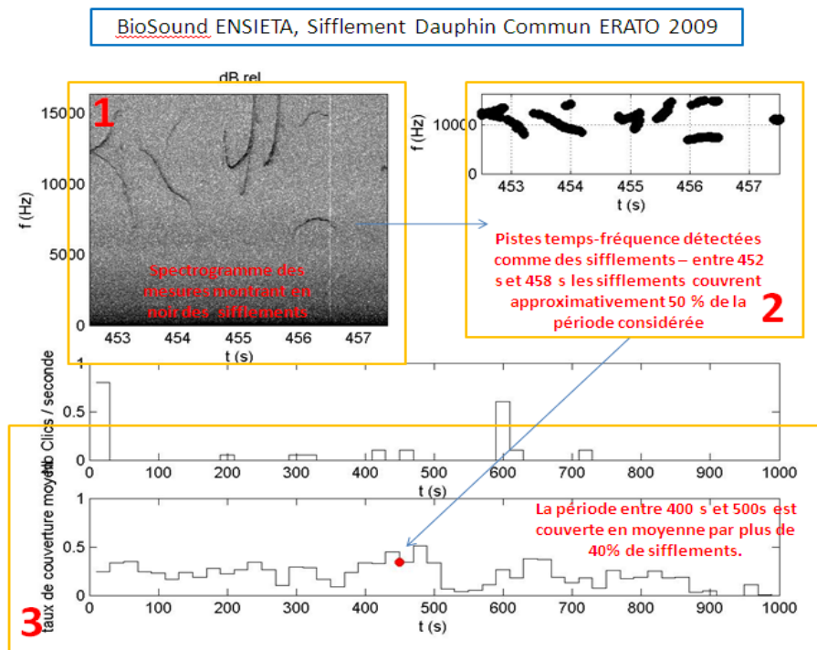
Figure 3 : Schéma de l'algorithme de détection. 1) spectrogramme du signal acoustique. Les « virgules » noires représentent des événements (sifflements) plus énergétiques que le bruit de fond (gris). 2) Les points noirs représentent des pixels énergétiques détectés, l'ensemble des pixels noirs dans la période d'analyse correspond au « taux de colonisation du spectrogramme ». 3) « Taux de couverture temporelle » après filtrage.
