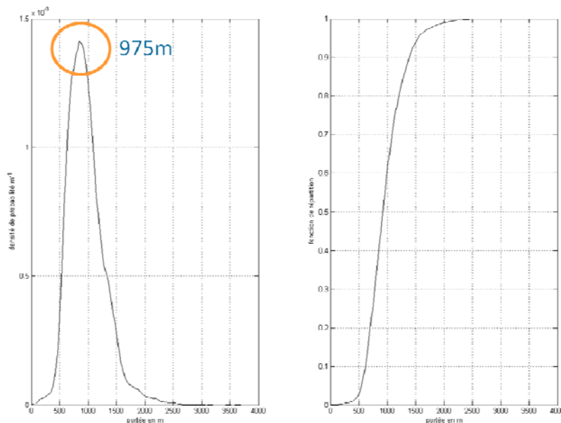
Figure 9 : Histogramme (gauche) et fonction de probabilité (droite) de la portée de détection d'un sifflement en BSO pour un système autonome ENSTA.
