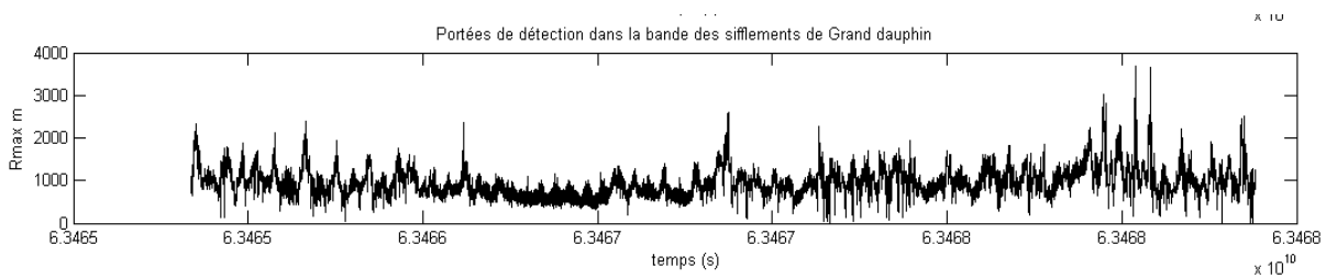
Figure 8 : Evolution de la portée de détection ( R_{max} , m) sur toute la période de l'enregistrement.
