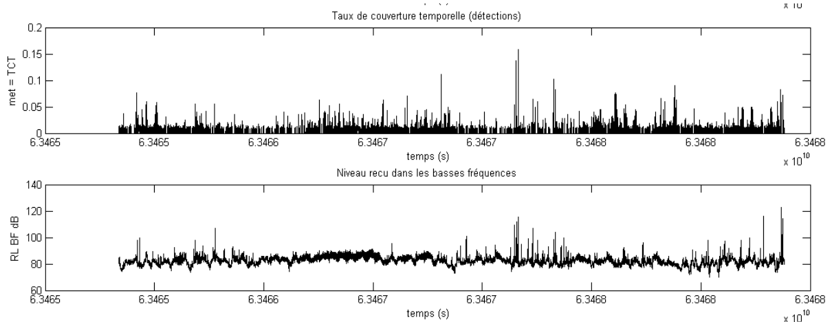
Figure 7 : En haut, taux de couverture temporelle (voir Fig. 4 & 5), en bas niveau reçu (dB) dans les basses fréquences (200-500 Hz).
