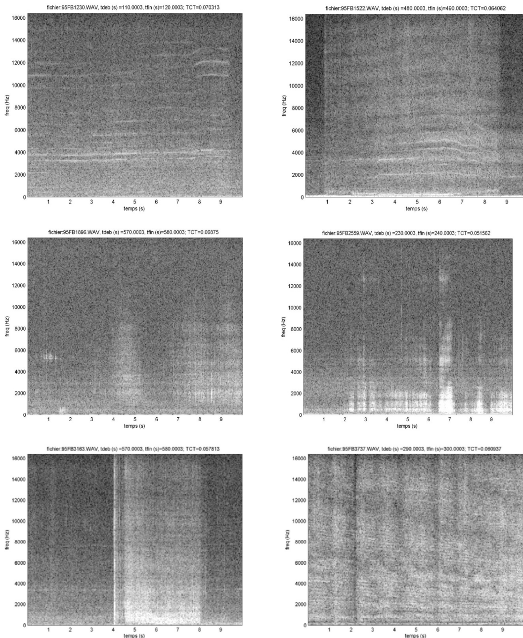
Figure 6 : Spectrogrammes de différents bruits détectés.
